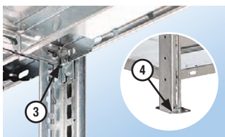
Fachbodenträger (3), Klemmfuß (4)
